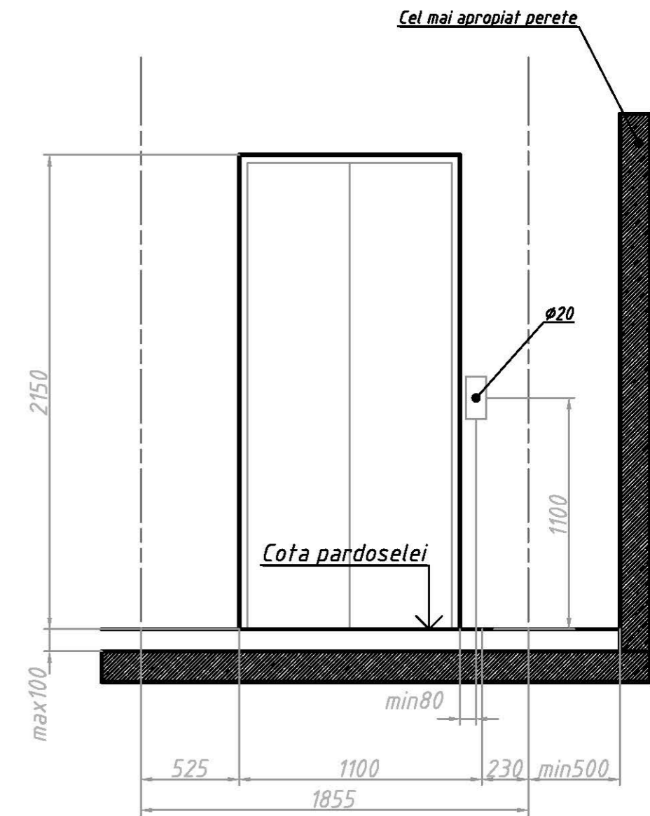
Etajele intermediare
